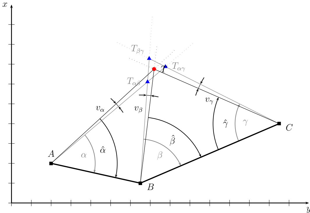
Slika 1–3: Prikaz metode najmanjših kvadratov pri določitvi koordinat točke T
