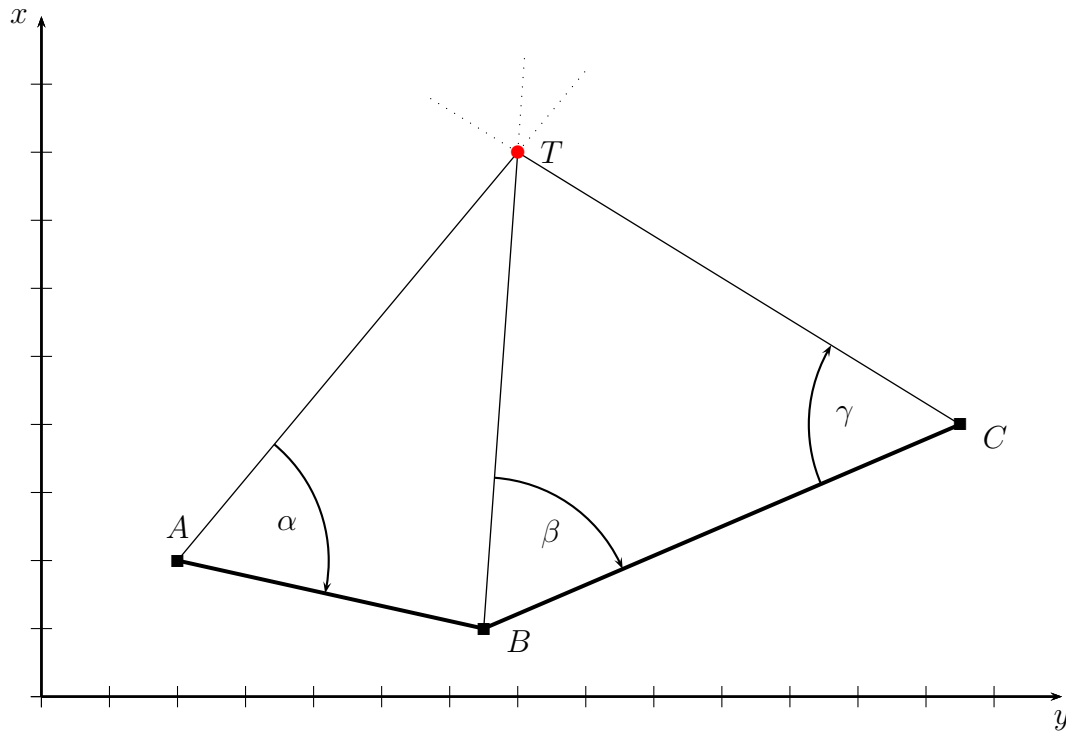
Slika 1–1: Prikaz podanih treh točk ( A , B in C ) in izmerjenih kotov ( \alpha , \beta in \gamma ) za določitev koordinat nove točke T
