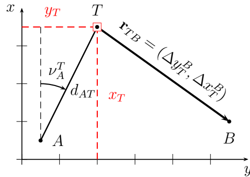
Slika 1-15: Izbiro neznank pri obravnavanju horizontalne geodetske mreže
