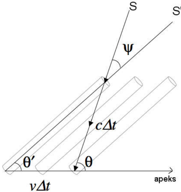
Slika 6: aberacija
