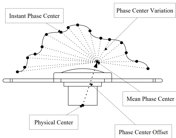
Slika 1: Konceptualni prikaz faznega centra GNSS-antene 9
