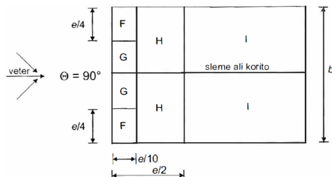
Slika 8: Shematski prikaz razdelitve dvokapnice po področjih pri delovanju vetra v smeri osi X
