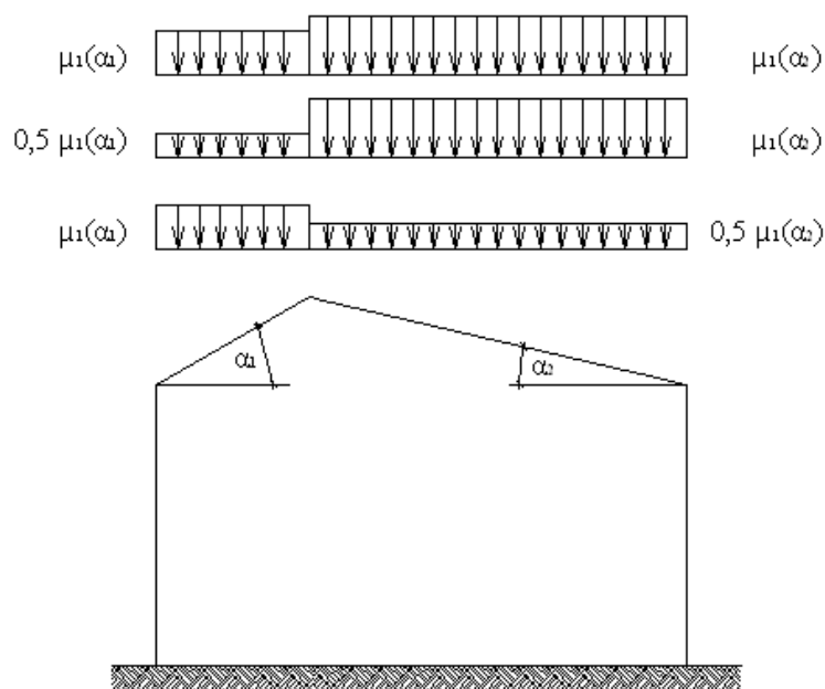
Slika 5 Oblikovni koeficienti obtežbe snega pri dvokapnici \mu(\alpha) .
