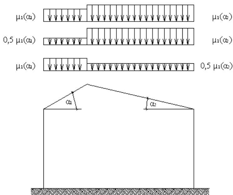
Slika 2 Oblikovni koeficienti obtežbe snega pri dvokapnici \mu_{\alpha_1} .
