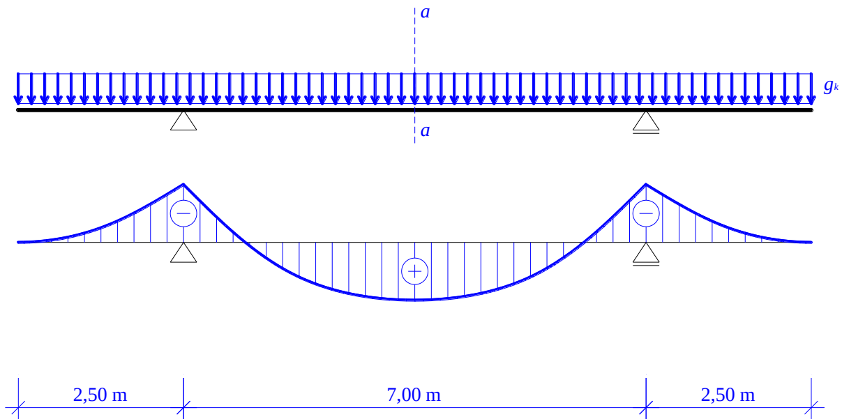
Slika 6 Stalna obtežba.
