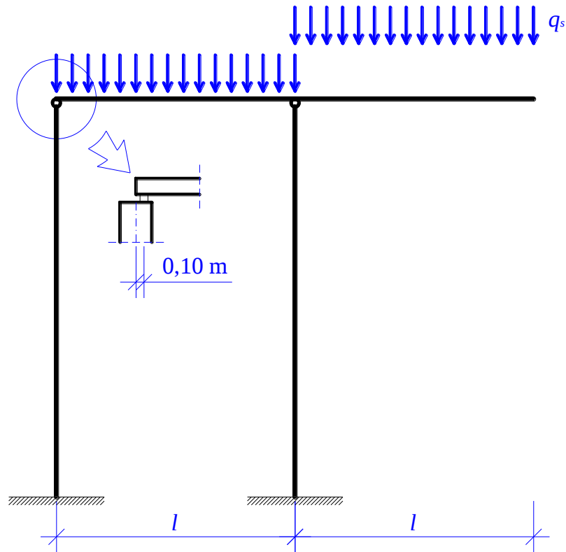
Slika 2 Statični model konstrukcije, v kateri se nahaja obravnavani steber.
