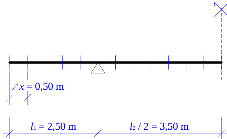
Slika 10 Model konstrukcije.
