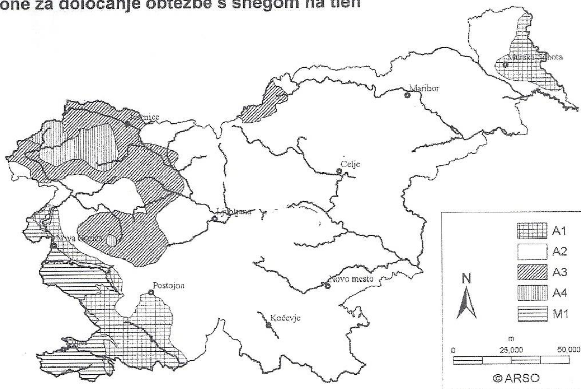
Slika 4 Obtežba snega na tleh.
