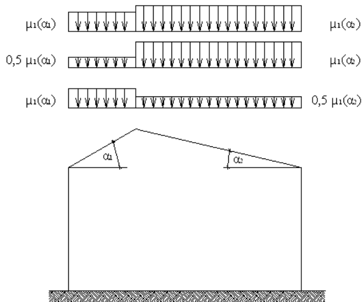
Slika 5 Oblikovni koeficienti obtežbe snega pri dvokapnici \mu(\alpha) .
