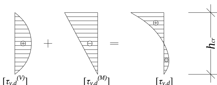
Slika 13 Potek tangencialnih (strižnih) napetosti.
