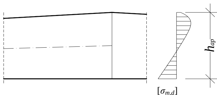
Slika 9 Potek normalnih napetosti v slemenu.
