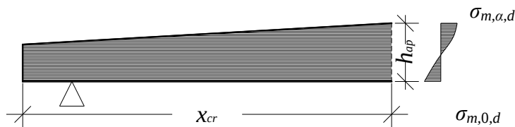
Slika 12 Potek normalnih napetosti v kritičnem prerezu.
