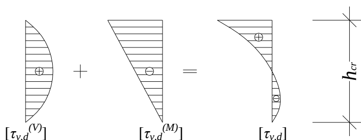
Slika 13 Potek tangencialnih (strižnih) napetosti.
