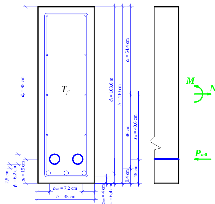
Slika 6 Notranje sile v prečnem prerezu.
