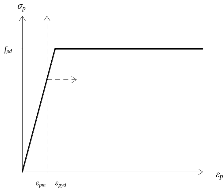
Slika 10 Delovni diagram jekla za prednapenjanje.
