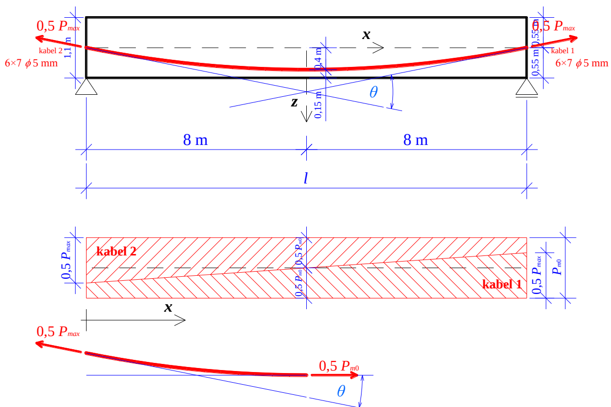
Slika 5 Potek kabske linije v prednapetem betonskem nosilcu in sila prednapetja.
