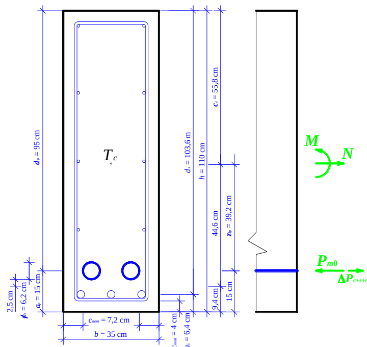
Slika 8 Padec sile prednapetja v kablh.
